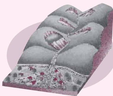
土石流による災害
