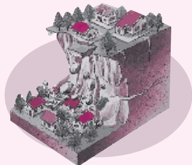
急傾斜地の崩壊による災害
