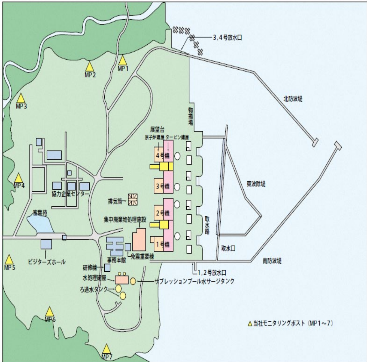
(1) 福島第二原子力発電所 配置図
