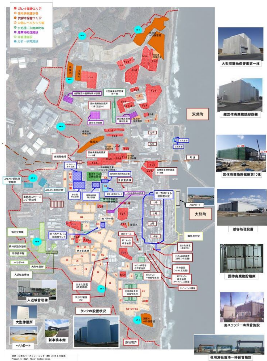
東京電力ホールディングス(株) 福島第一原子力発電所 配置図
