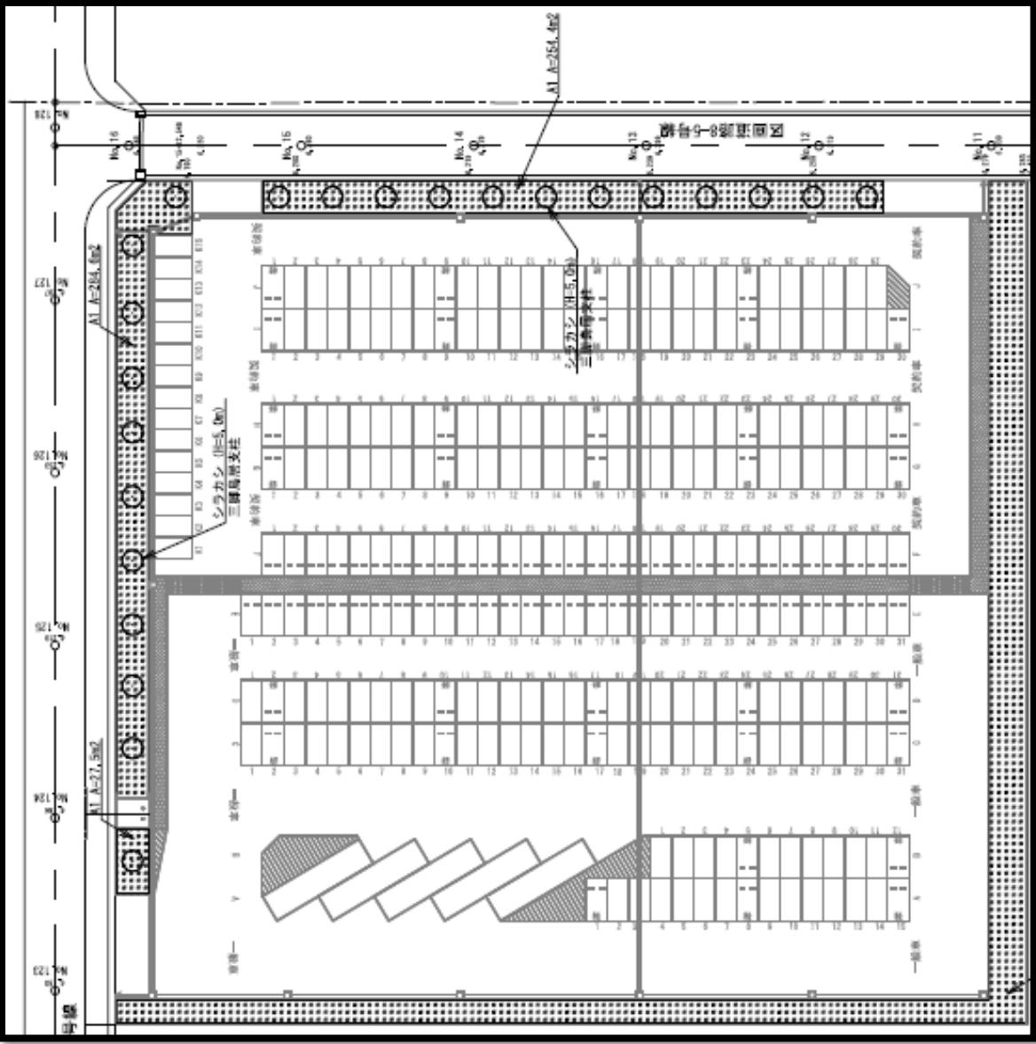
別添資料 1 寸法図 3 (南駐車場)
