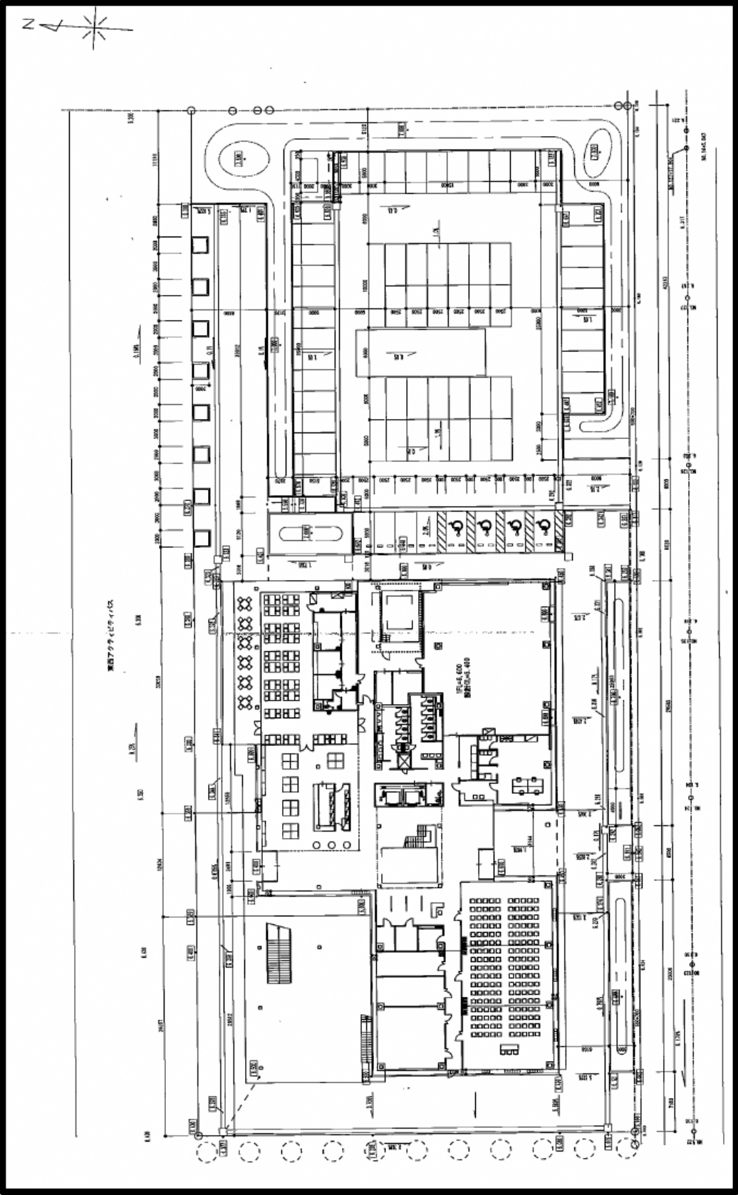
別添資料 1 寸法図 1 (本体及び東駐車場)
