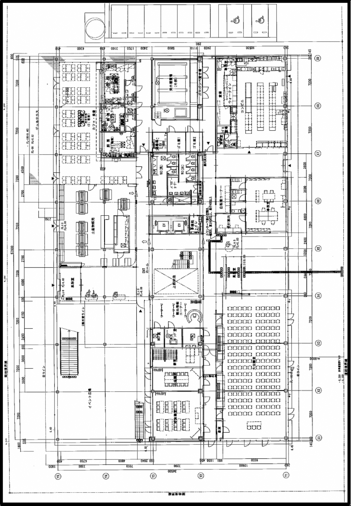
別添資料 1 居室概要等「1階平面図」
