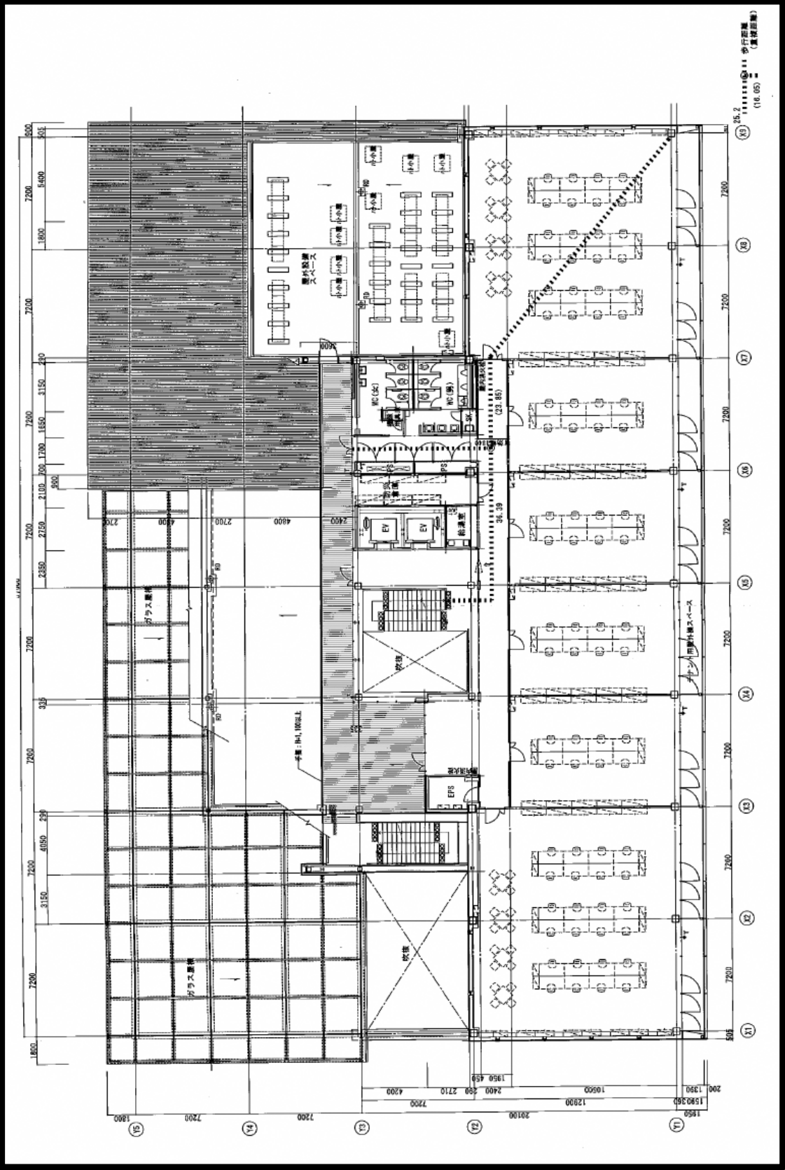
別添資料 1 居室概要等「3階平面図」
