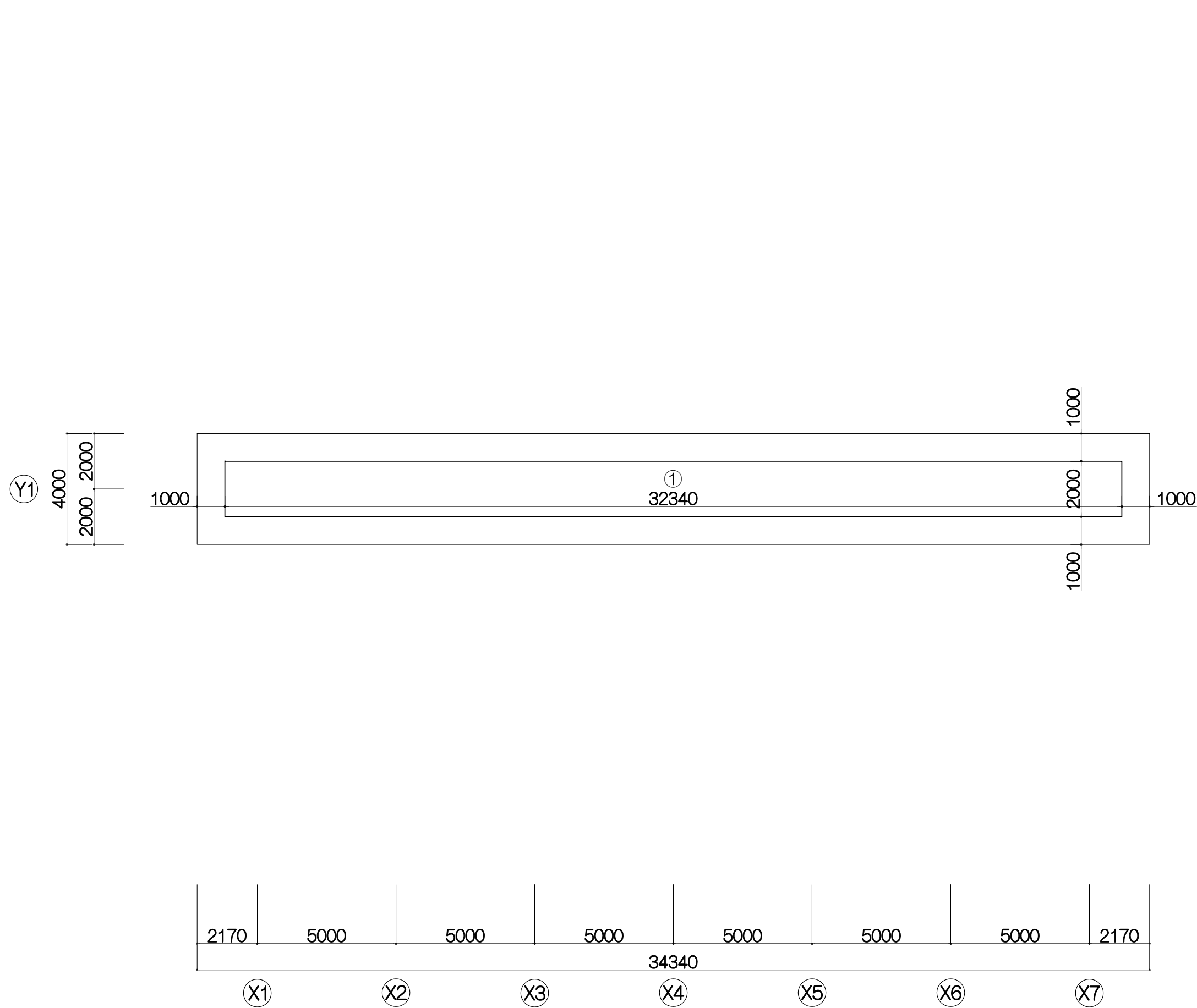
付帯施設D_求積図
