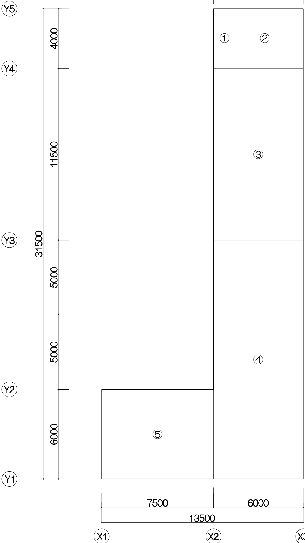
付帯施設B_求積図
