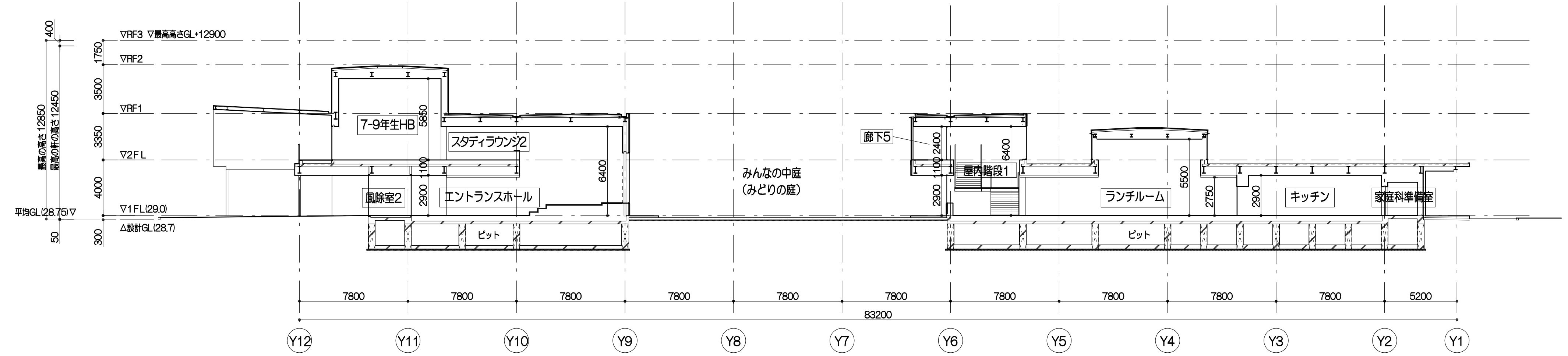
E-E' 断面図
