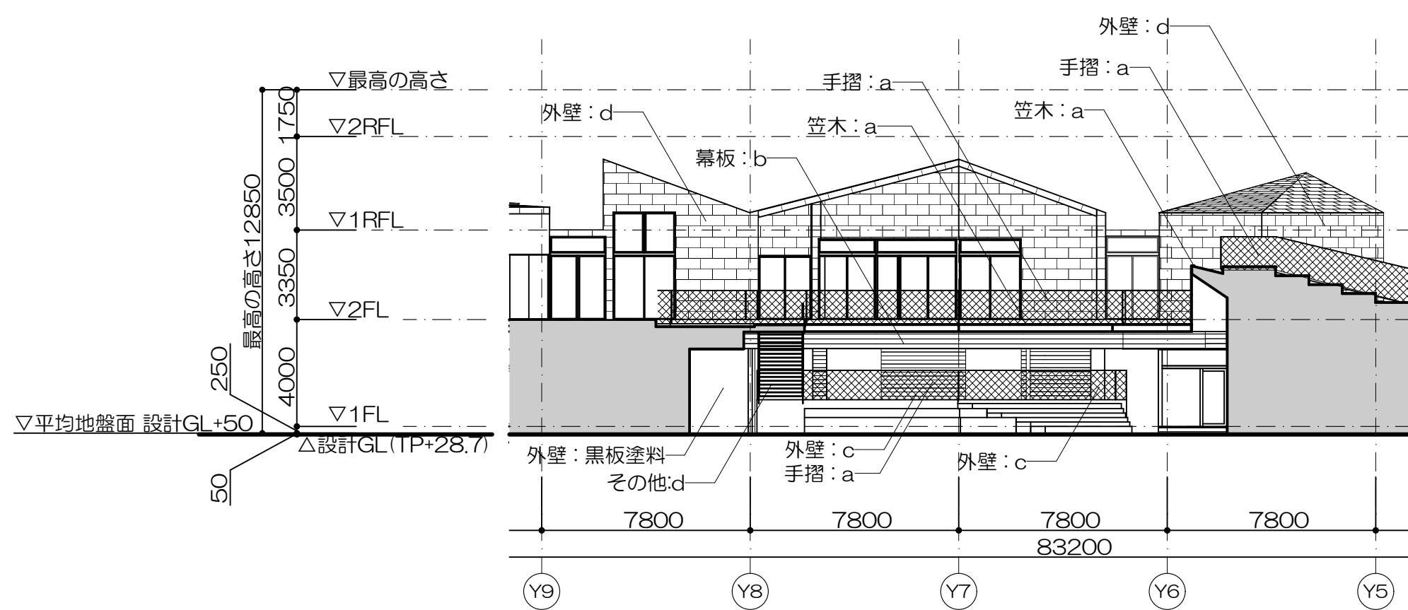
中庭 中央通路面 F立面図
