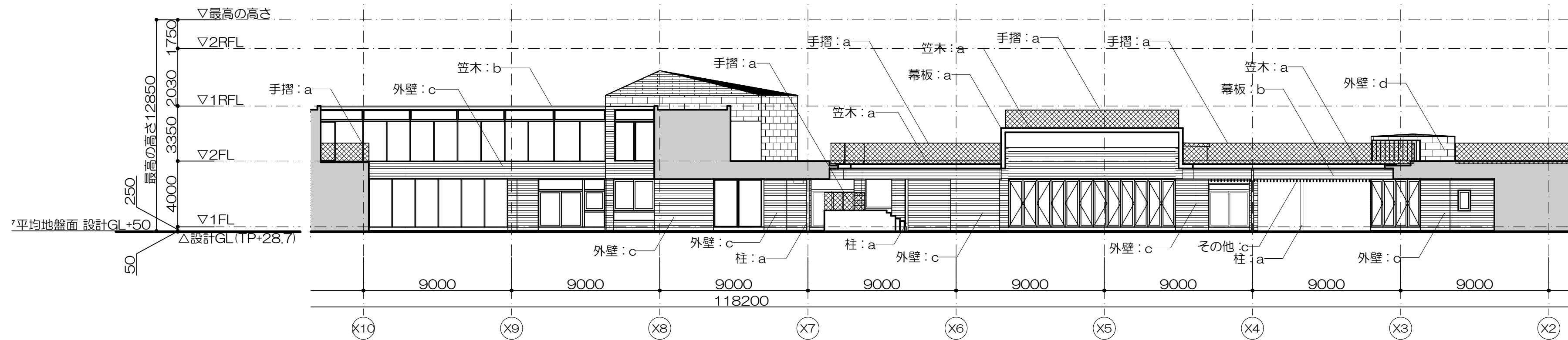
中庭 B立面図
