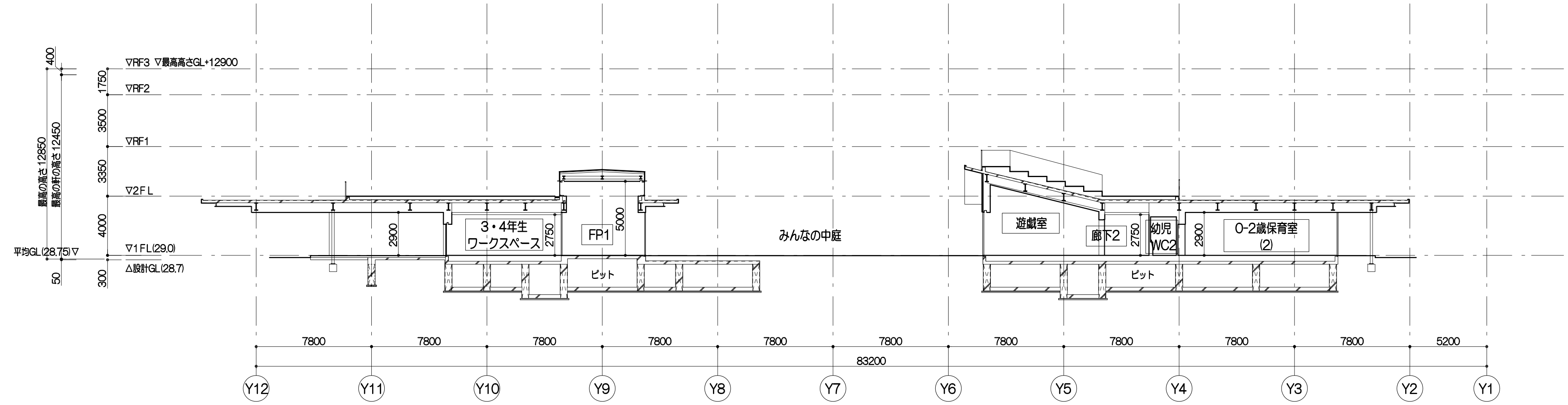
C-C' 断面図
