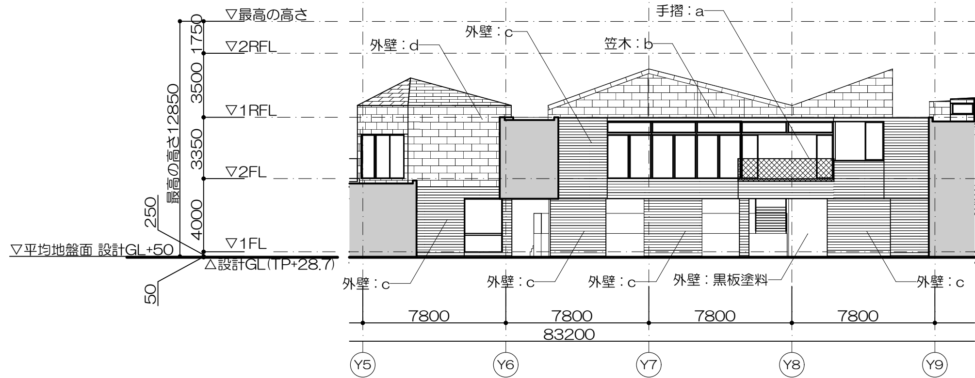
中庭 中央通路面 E立面図
