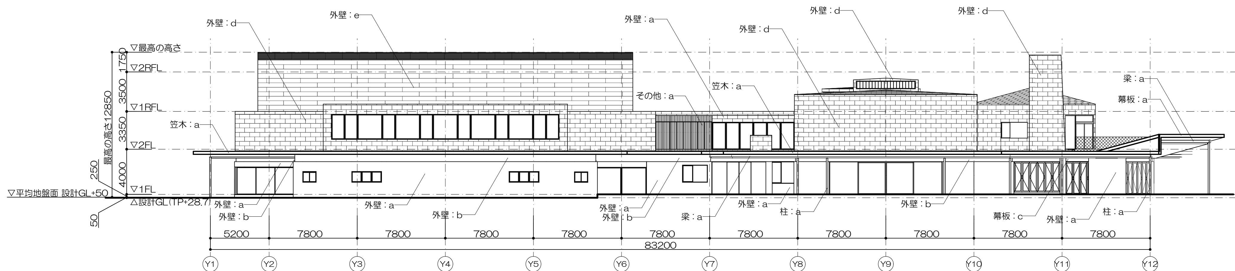
東立面図
