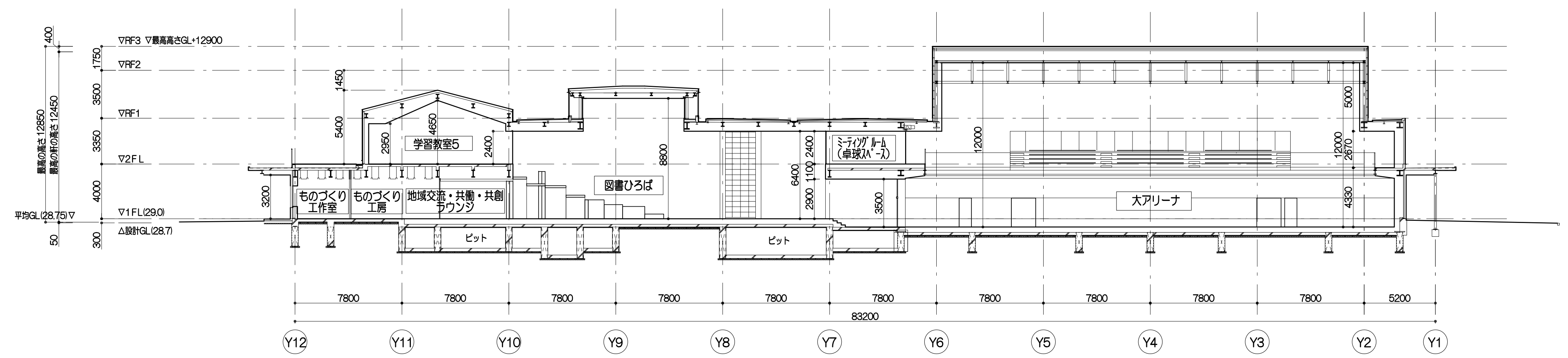
F-F' 断面図
