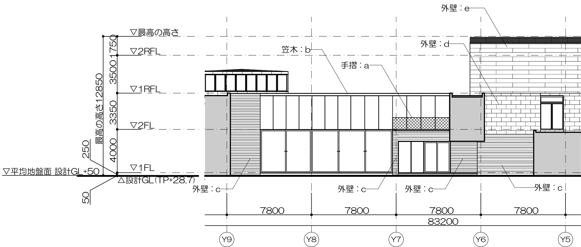
中庭 D立面図
