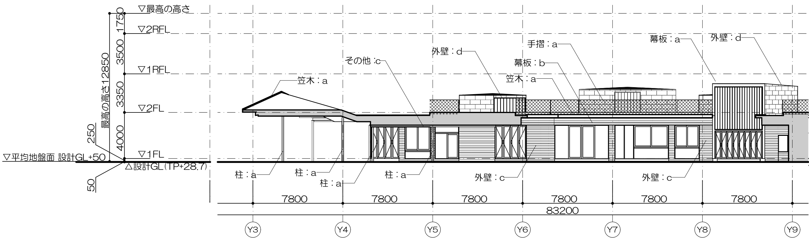
中庭 C立面図
