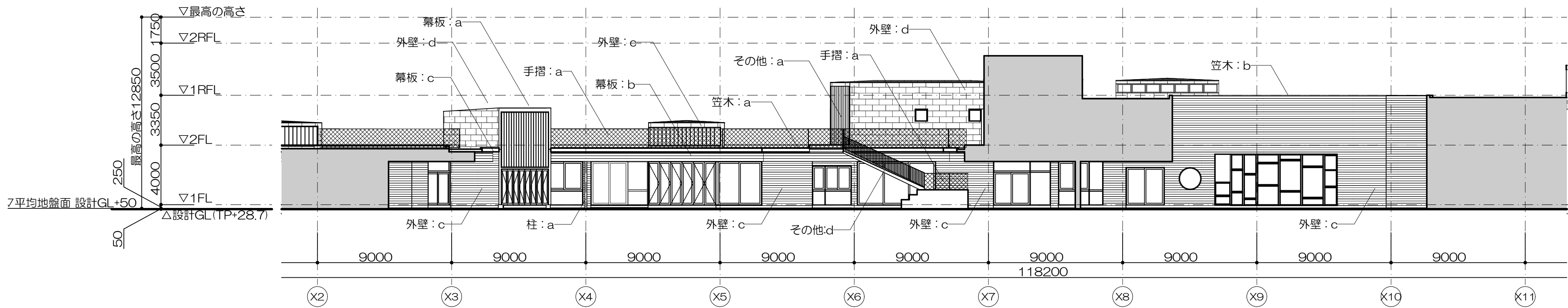
中庭 A立面図
