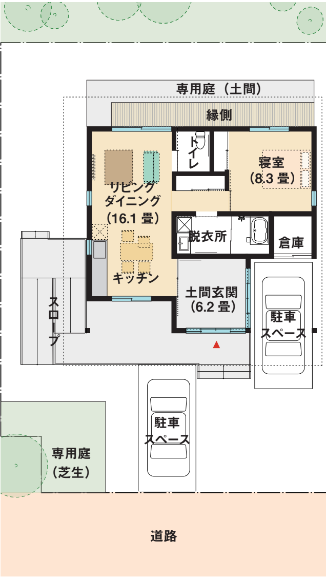
1階平面図
